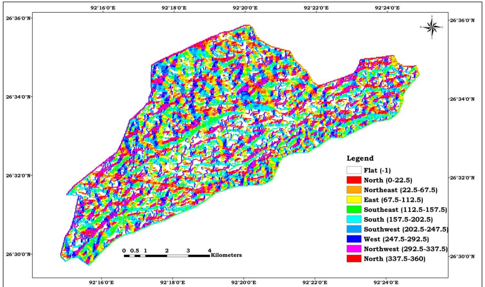
Fig. I f) - Aspect Map of RG Orang NP
