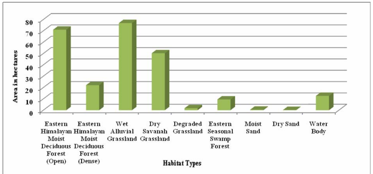
Fig. V r) Habitat pattern of Tinkona Block
