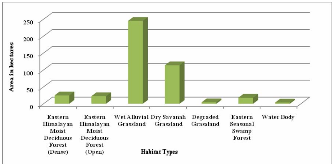
Fig. V p) Habitat pattern of Satsimalu Block
